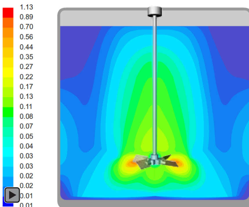
Análisis de dinámica de fluidos computacional del álabe E-400
